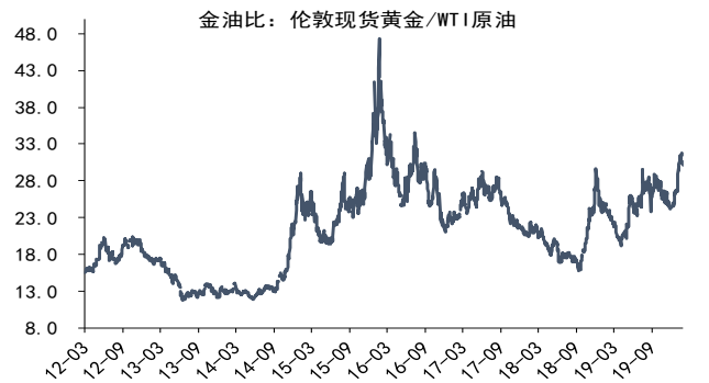
图 16: 金油比
