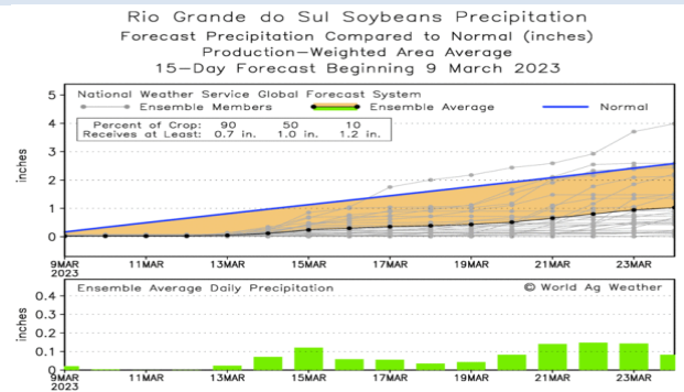
图4 未来15天巴西南里奥格兰德州降雨
