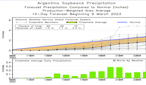
图5 未来15天阿根廷大豆产区降雨
