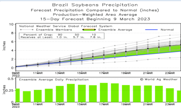
图3 未来15天巴西大豆产区降雨
